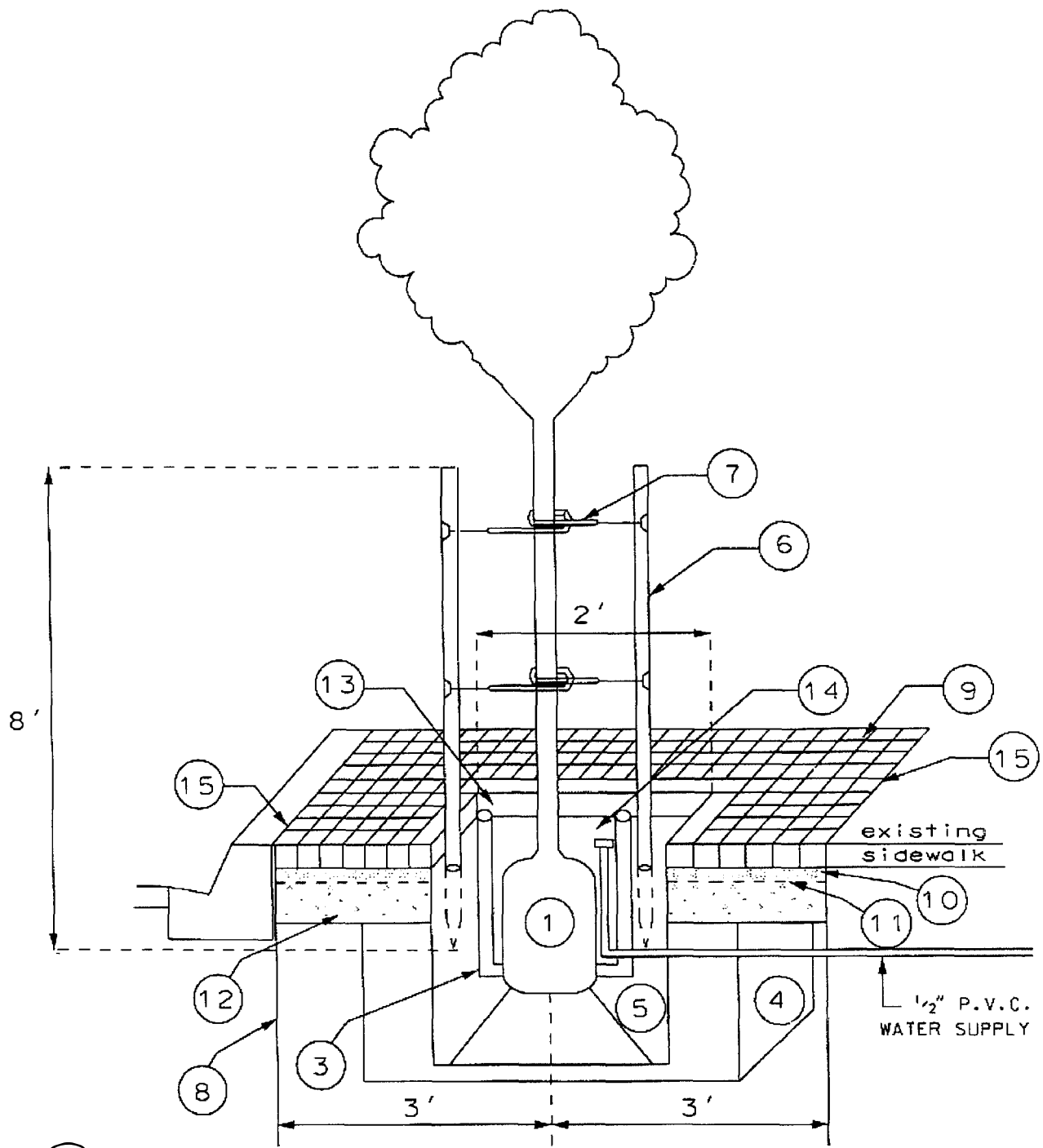
SECTION A-A
